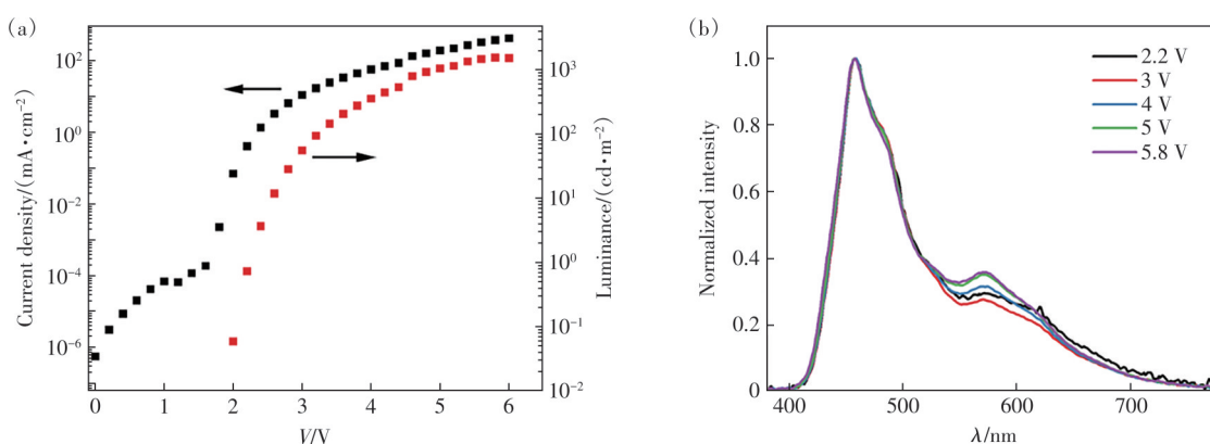
图3 低开启电压蓝光TTA上转换有机发光二极管的电致发光特性。(a)电流密度-亮度-电压特性;(b)不同电压下高于开启电压的电致发光光谱
