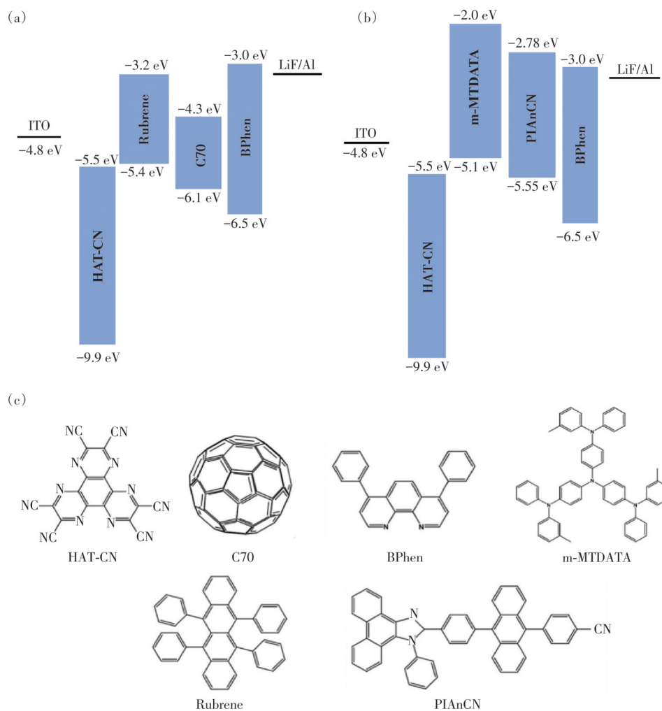
图1 橙光(a)与蓝光(b)TTA上转换OLED器件结构示意图;(c)有机材料的分子结构
