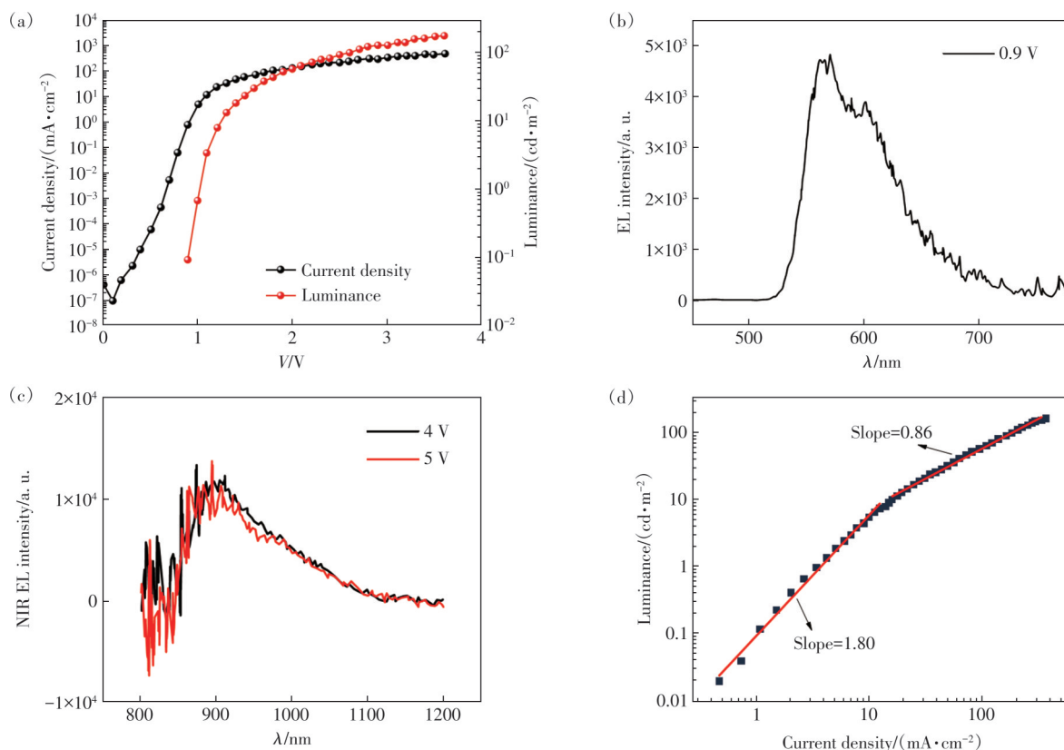
图 2 低开启电压橙光 TTA 上转换 OLED 的电致发光特性。(a) 电流密度-亮度-电压特性;(b) 0.9 V 电压下的电致发光光谱;(c) 4 V 和 5 V 电压下的电致发光光谱;(d) 亮度-电流密度特性
